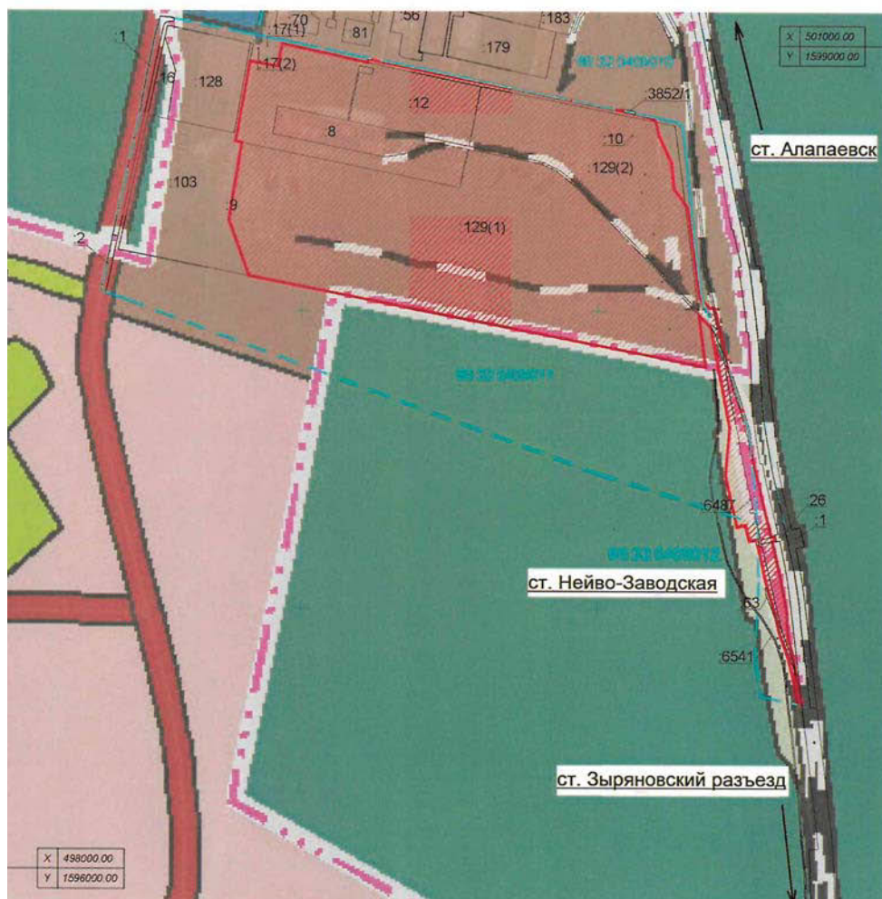
Схема границ территории, в отношении которой осуществляется подготовка документации по планировке территории для размещения линейного объекта «Железнодорожная инфраструктура необщего пользования для комплекса по производству мелющих стальных шаров»
